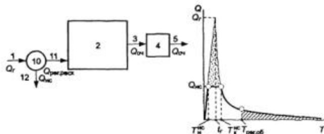
Рис. 2. Схема перекачки избыточной части зарегулированного по объему дождевого стока
