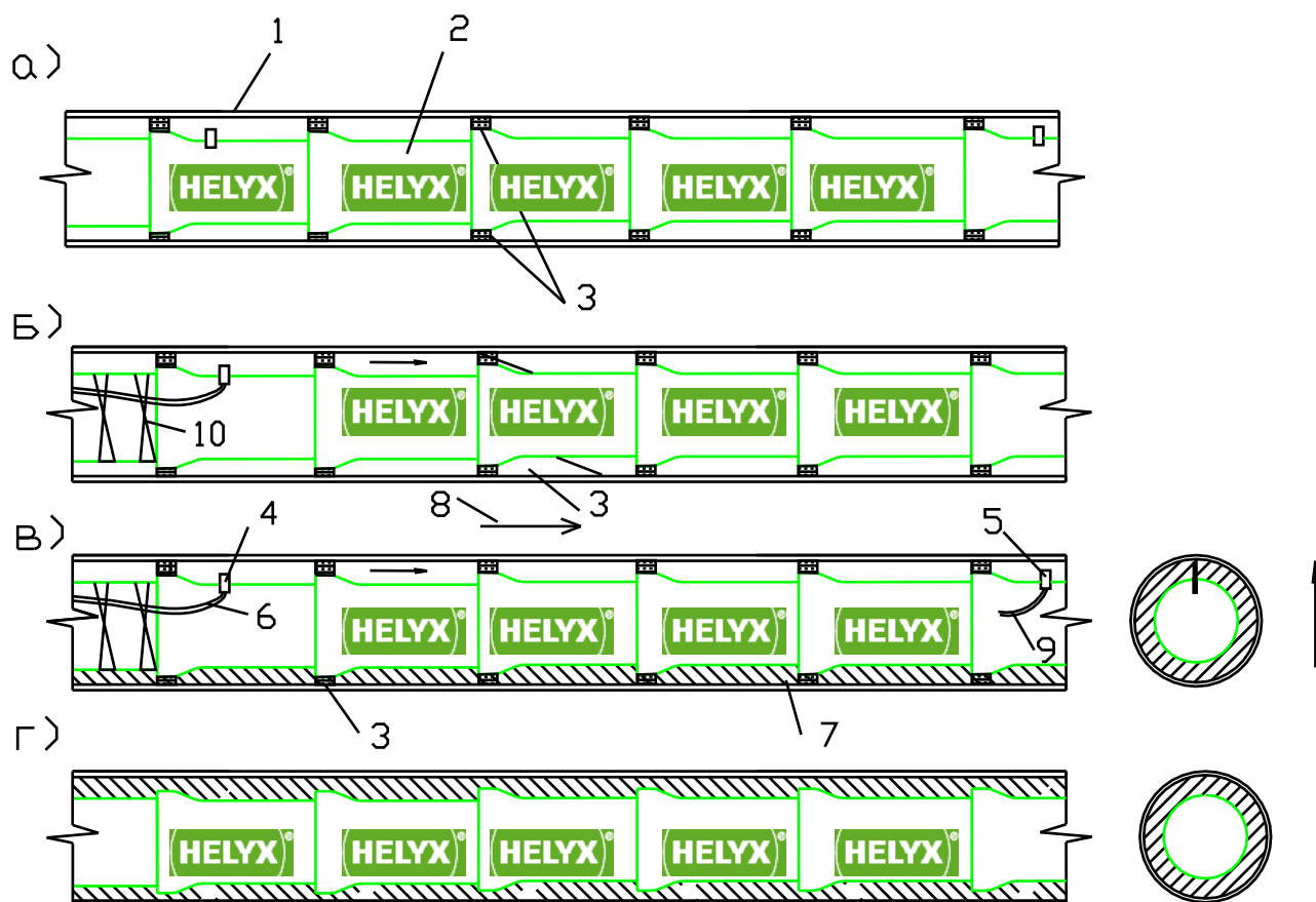
Рис. 37 Заполнение межтрубного пространства цементно-песчаным раствором (2 способ)
