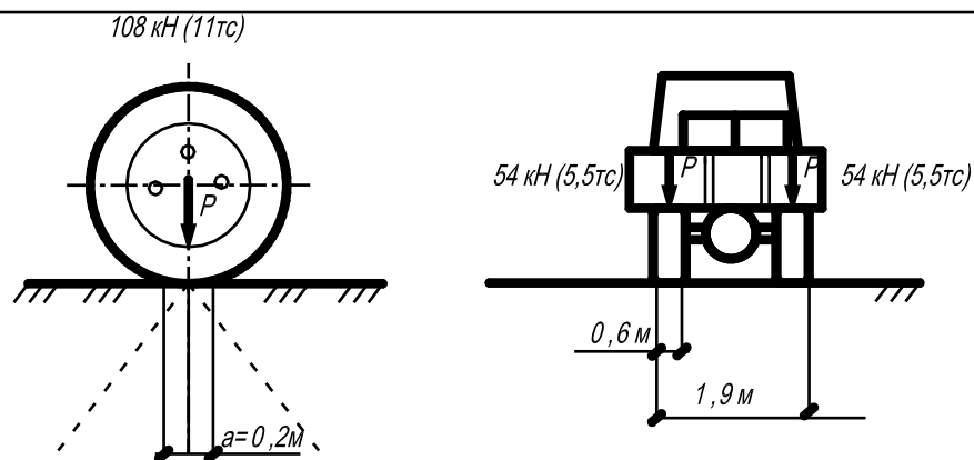
Рис 8 Колесная нагрузка от одноосной тележки с давлением 108 кН (11 тс).
