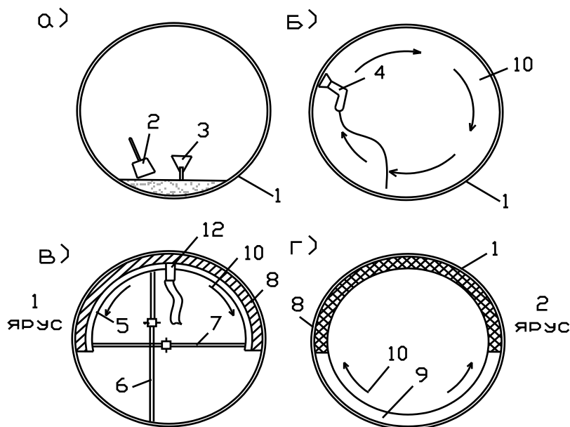
Рис. 22 Подготовка существующей ж/б трубы к санации
