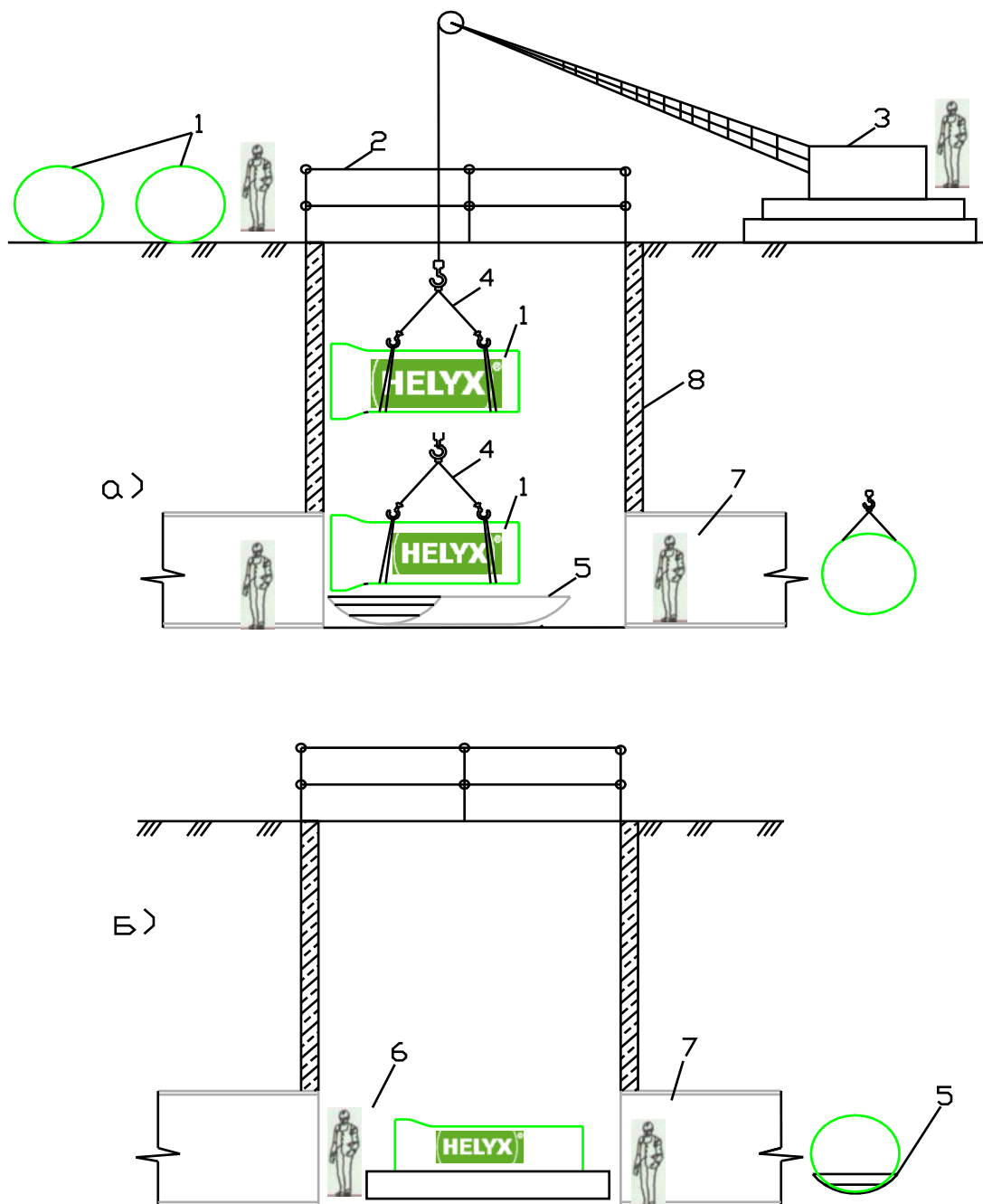
Рис 26 Установка трубы HELYX на корыто
