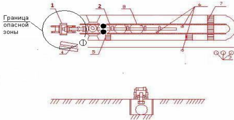
Рис.50. Схема производства работ по укладки стеклопластиковых труб
