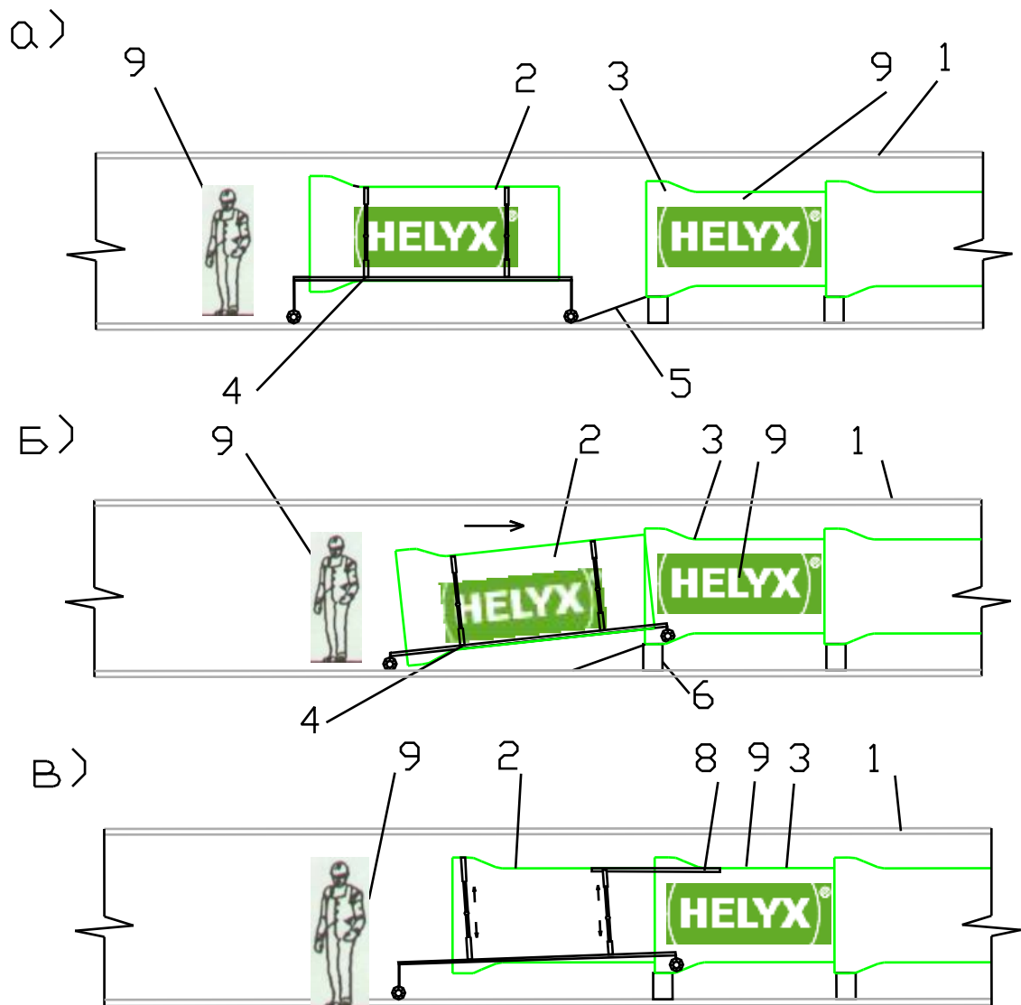
Рис. 29 Установка трубы на месте монтажа с использованием тележки
