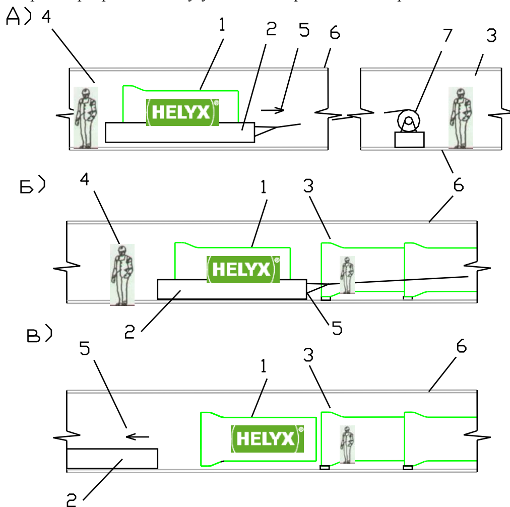
Рис. 27 Транспортировка трубы HELYX к месту установки с использованием лебедки
