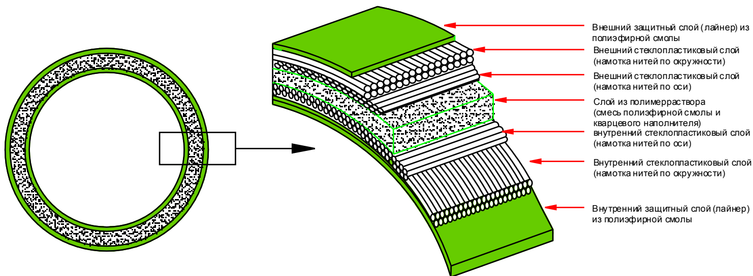
Рис.1 Разрез стеклопластиковой трубы Helyx.
