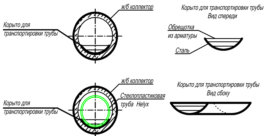
Рис 24 Корыто для транспортировки труб
