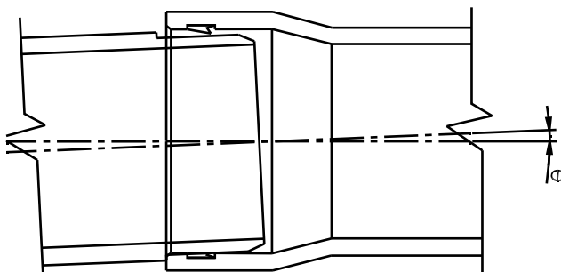
Рис 19. Угол изгиба (угловое смещение) в соединении
