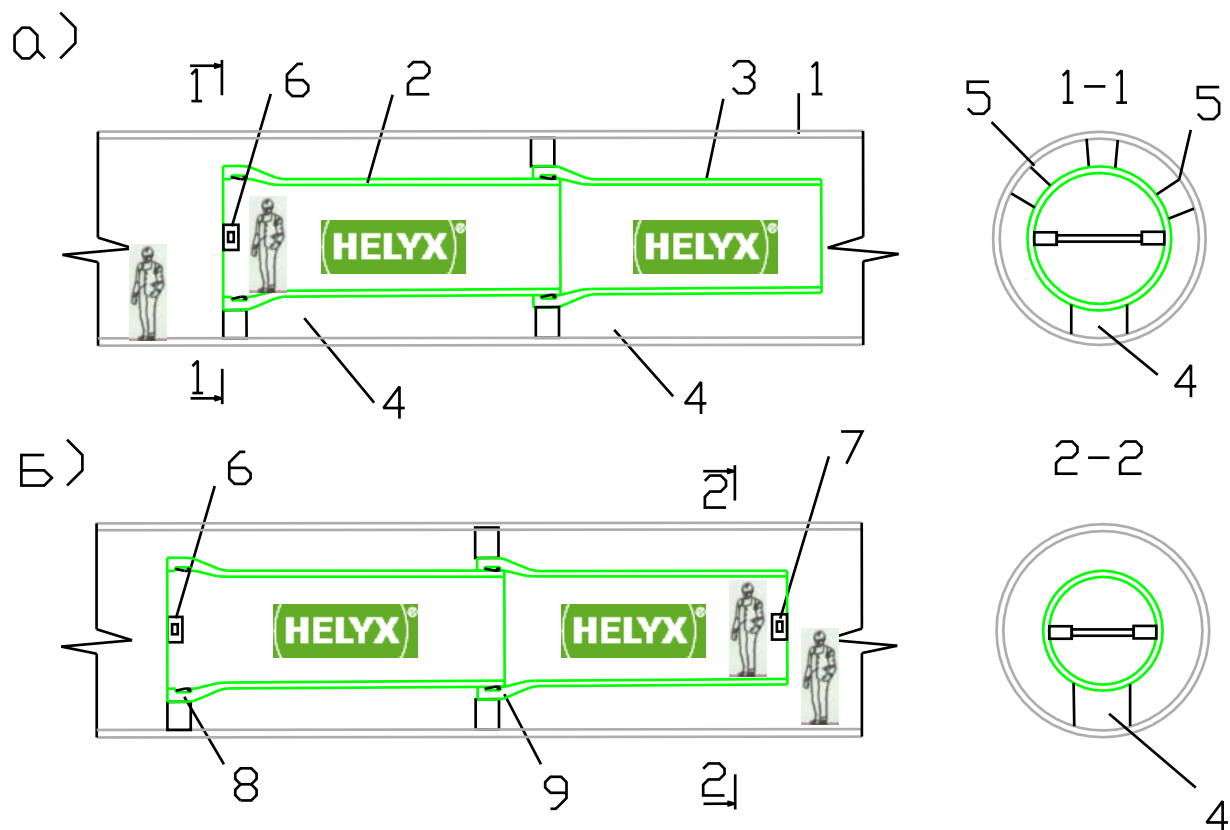
Рис.30 Установка монтажных распорок
