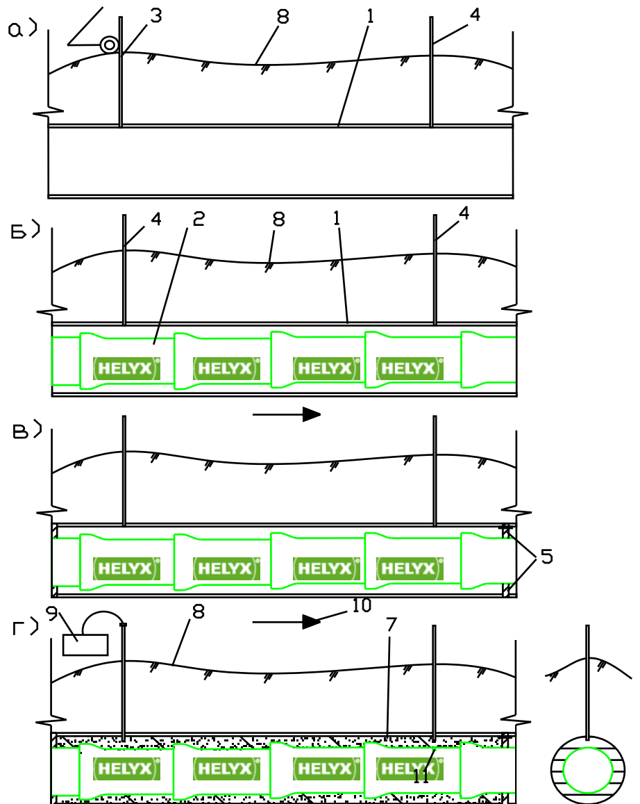
Рис. 36 Заполнение межтрубного пространства цементно-песчаным раствором (1 способ)
