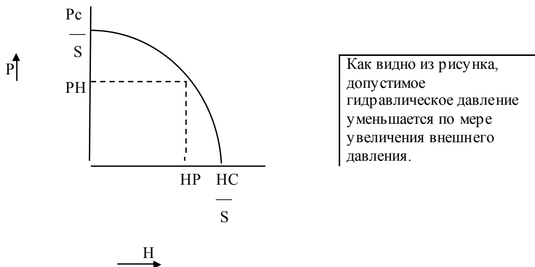
Рис. 11. Зависимость допустимого гидравлического давления от линейной нагрузки
