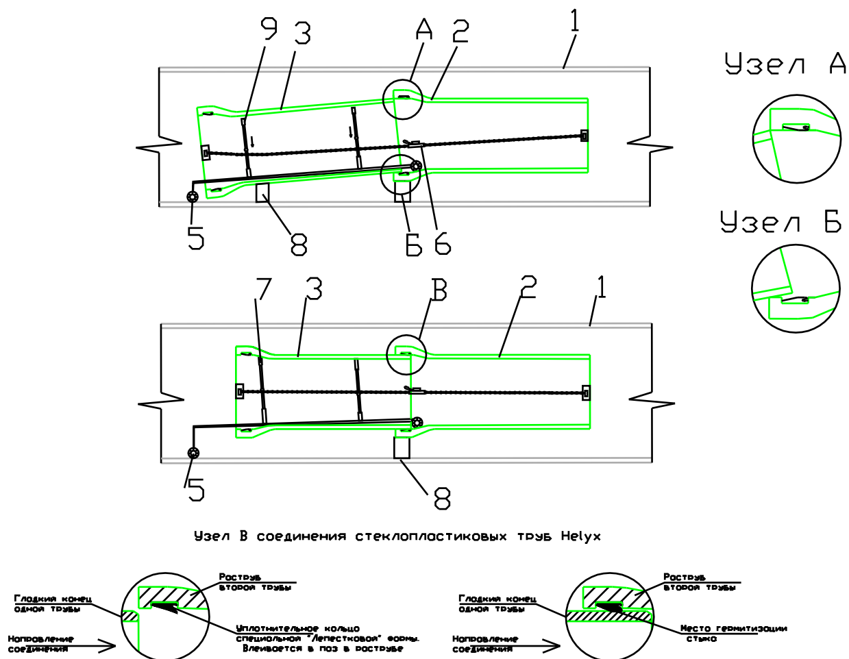
Рис.32 Установка труб HELYX с изменением уклона
