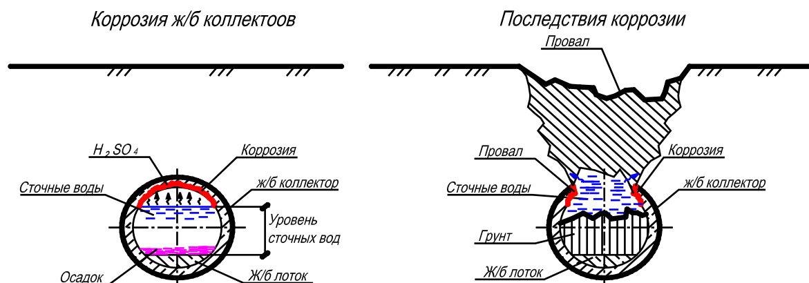
Рис 21 Коррозия бетонных труб
