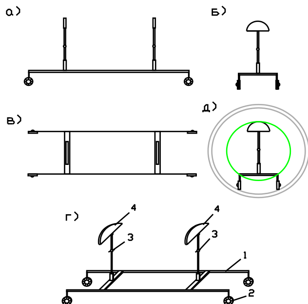
Рис. 23 Тележка для транспортировки и установки труб а) вид спереди б) вид сбоку, в) вид сверху г) пространственная модель д) вид тележки в трубе 1 – металлическая труба 2 – колеса на пневмоходу 3 – реечный домкрат усилием 2т 4 – упоры
