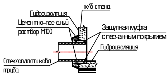
Заделка труб в мокрых грунтах
