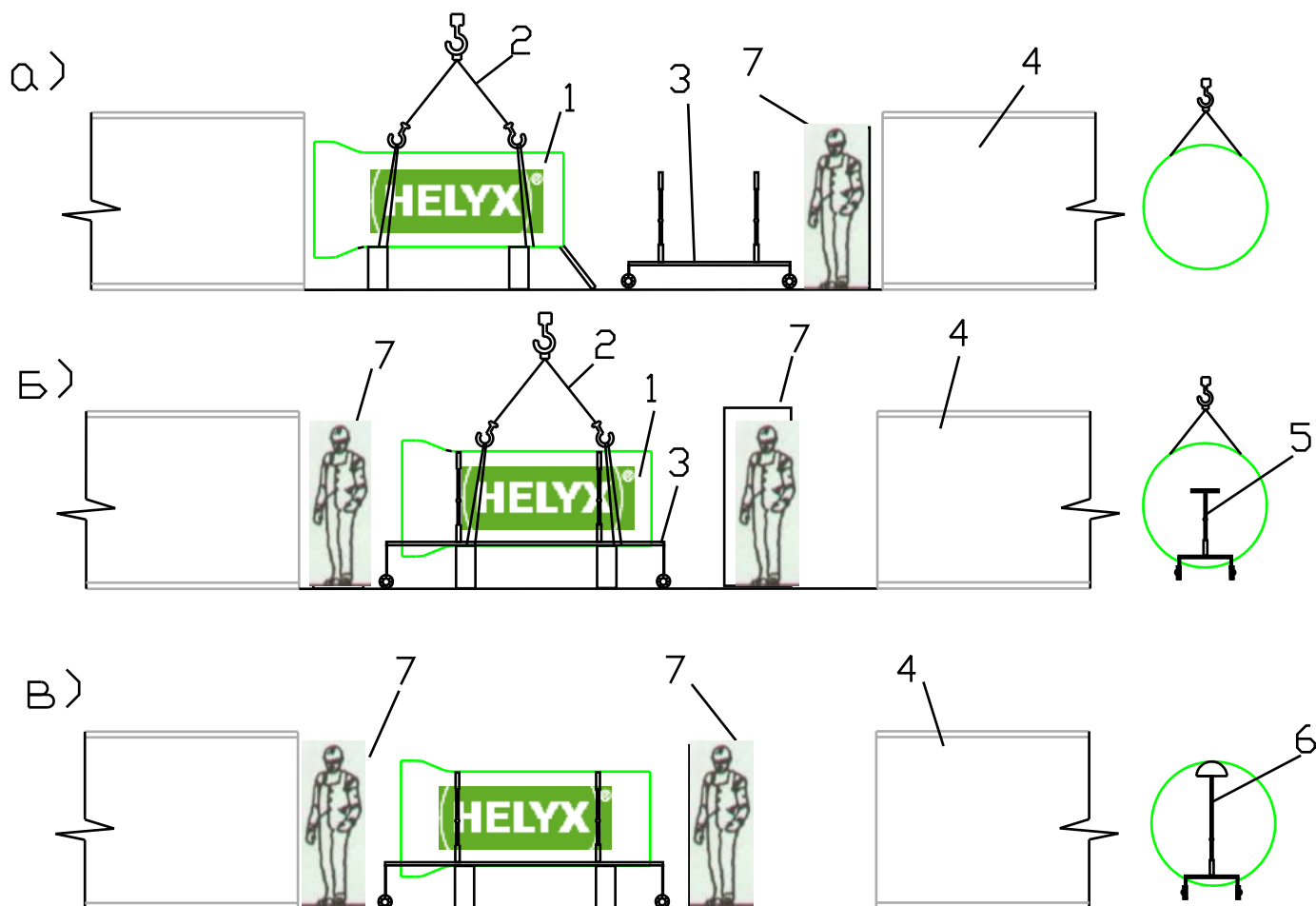
Рис.25 Установка трубы HELYX на тележку
