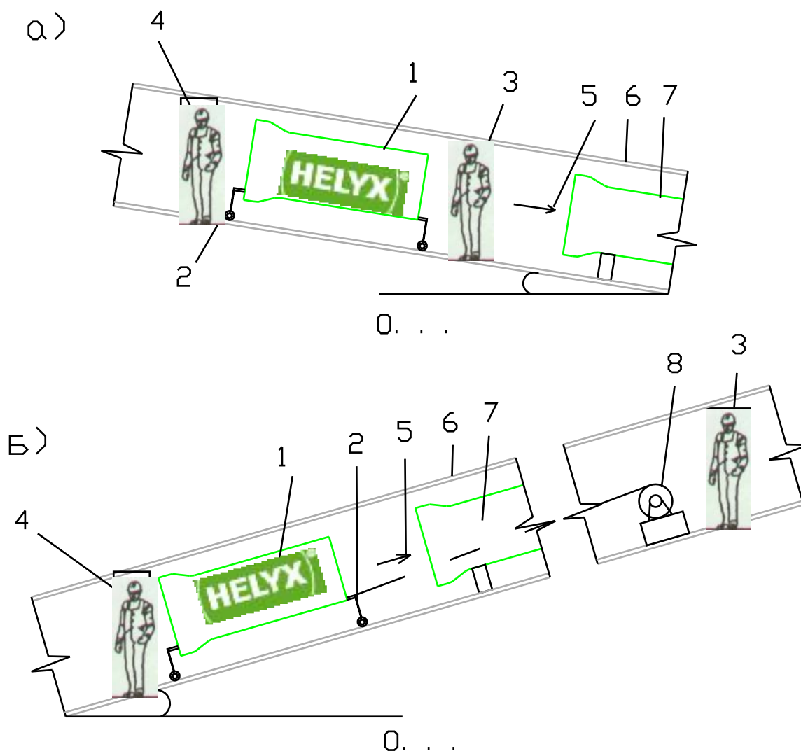
Рис. 28 Транспортировка трубы HELYX к месту установки
