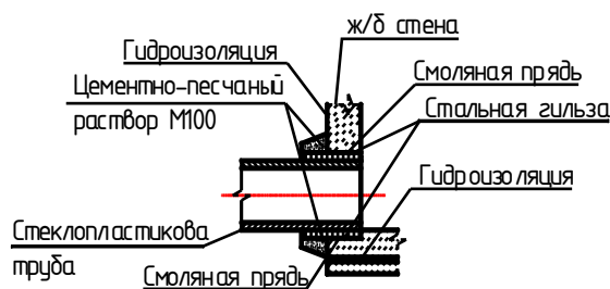
Заделка труб в мокрых грунтах
