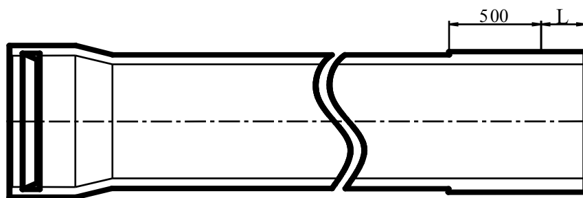
Рис.54. Регулировочная труба
