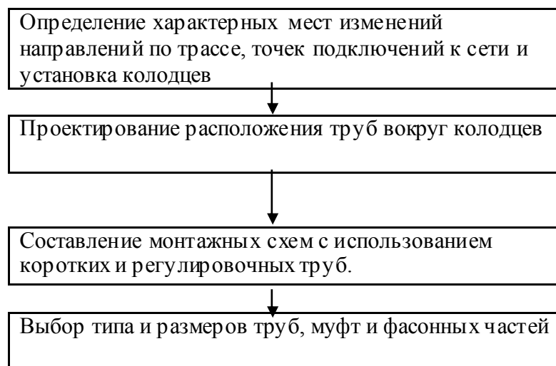
Рис 13 Алгоритм проектирования с применением стеклопластиковых труб.
