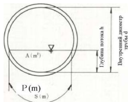
Рис 4. Сечение трубопровода
