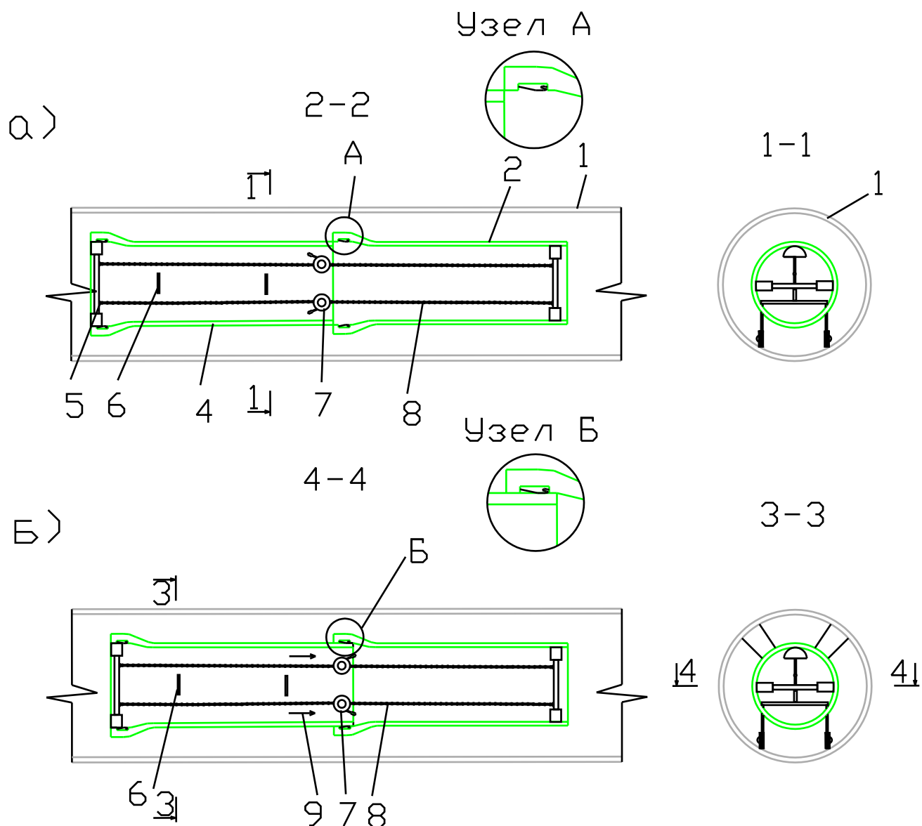
Рис.31 Соединение труб HELYX (соосно)
