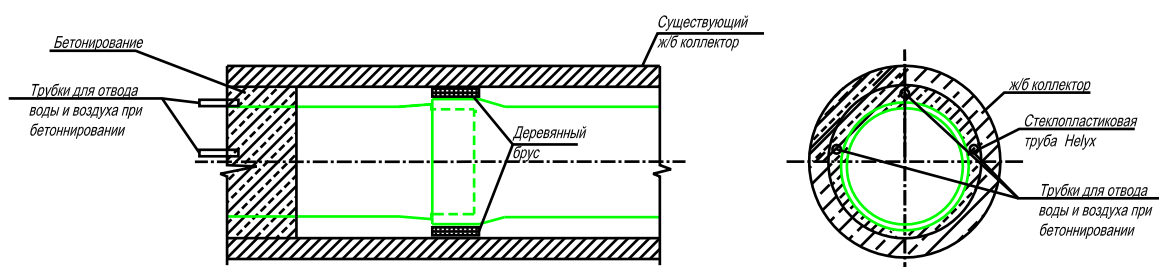
Рис 35 Бетонирование концов коллектора
