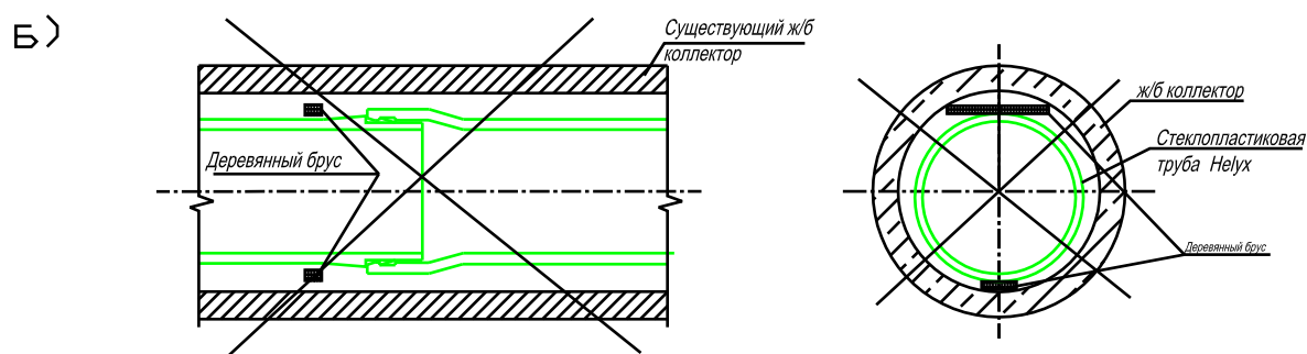
Рис 34 Установка деревянных подкладок для центровки трубы.
