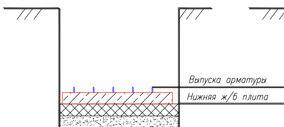
Нижняя ж/б плита
